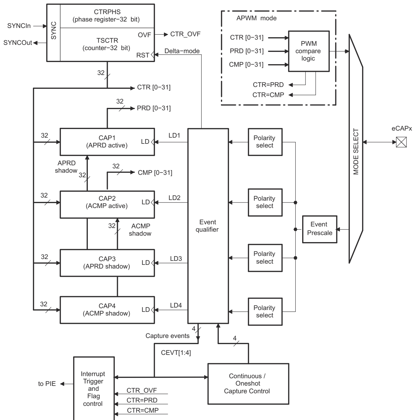
图 6-53. eCAP 方框图
