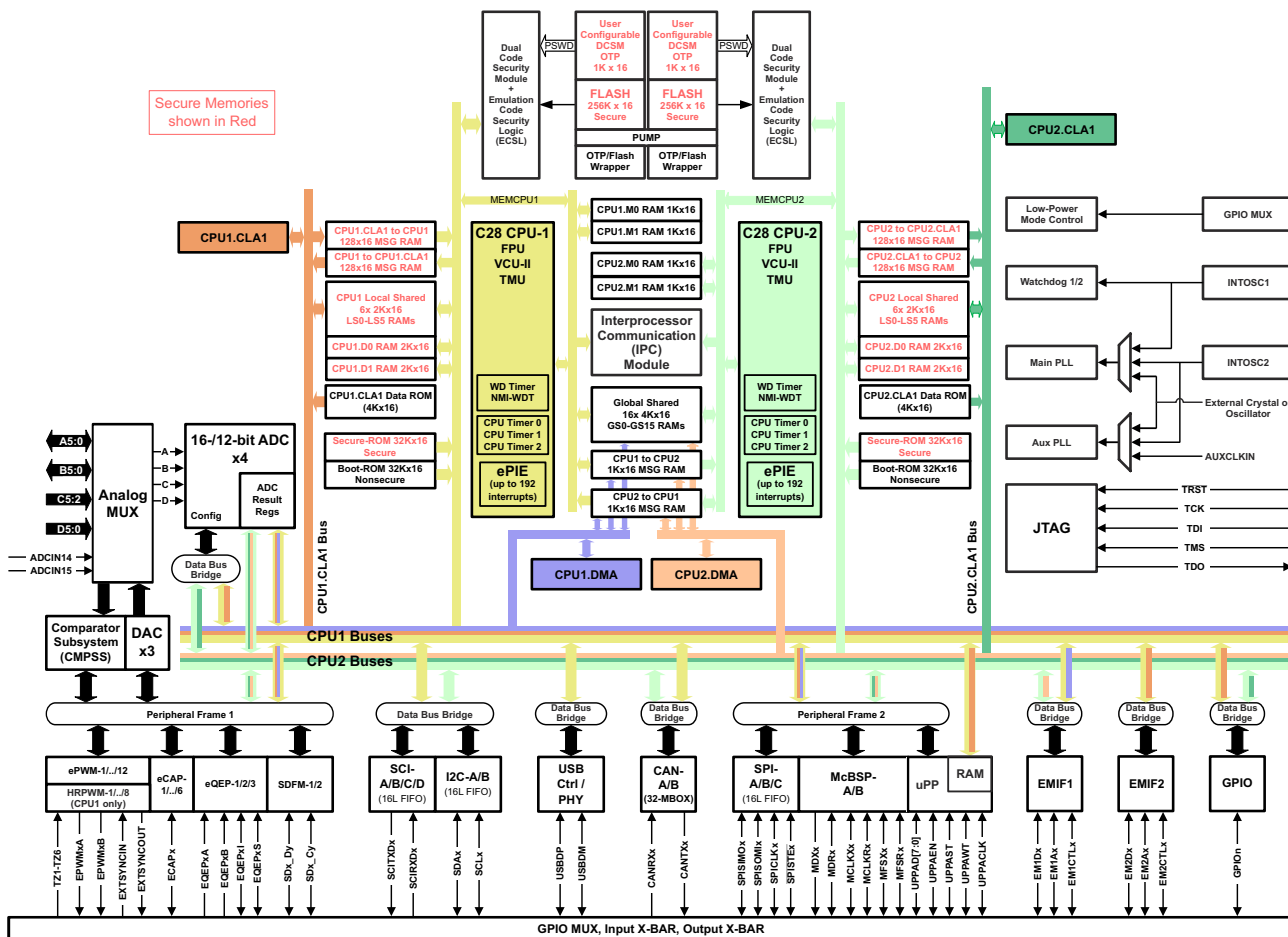
图 7-1. 功能方框图
