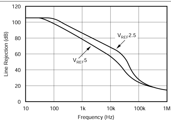
图 5-19. 参考交流线路抑制与频率间的关系
