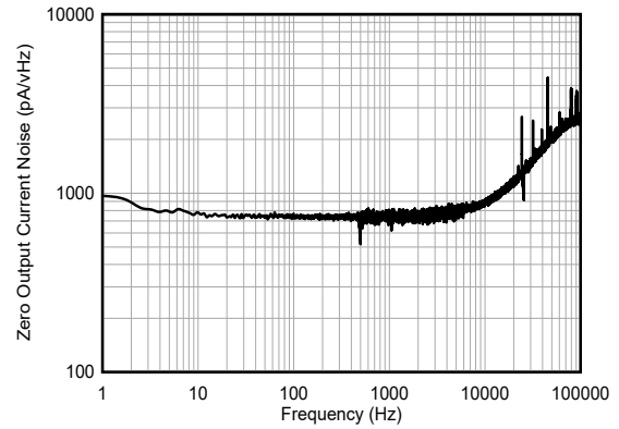
图 5-14. 零输出电流噪声密度与频率间的关系
