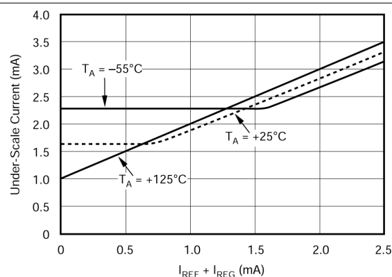
图 5-8. 欠量程电流与 I_{\text{REF}} + I_{\text{REG}} 间的关系
