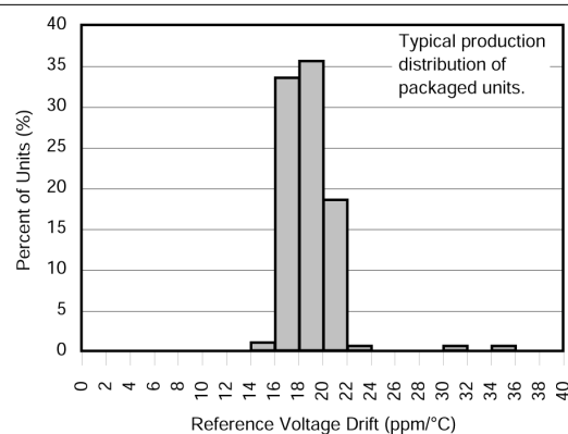
图 5-20. 参考电压漂移产生分布
