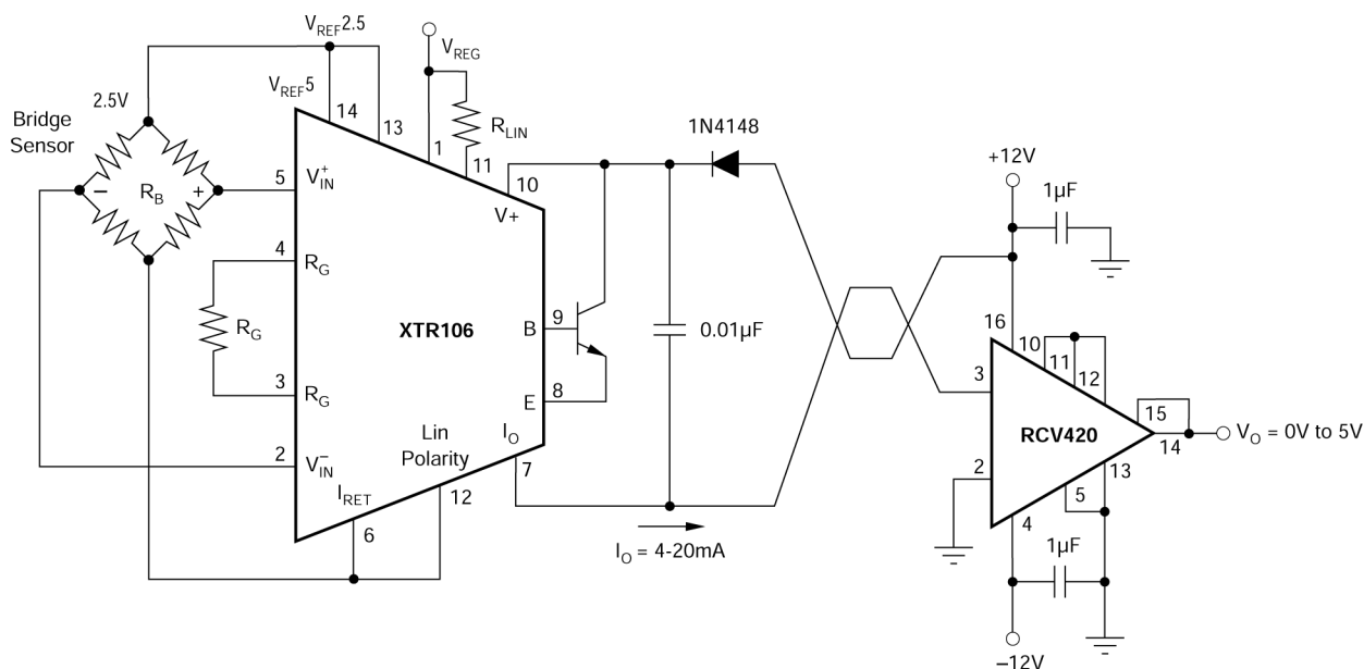
图 7-6. 由 ±12V 供电的发送器和接收器环路
