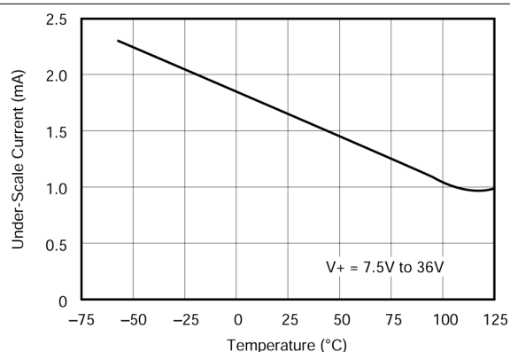
图 5-7. 欠量程电流与温度间的关系
