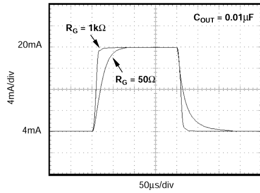
图 5-2. 阶跃响应
