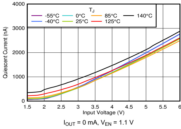
图 6-9. I_Q vs V_{IN} and Temperature
