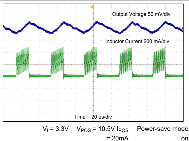
图 8-11. Boost Converter ( V_{POS} ) Output Ripple
