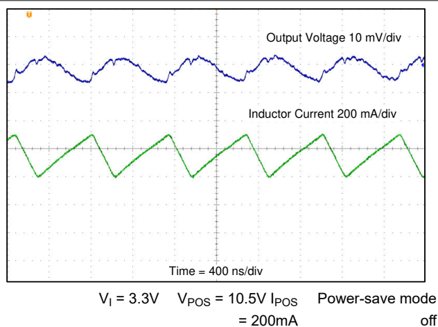
图 8-10. Boost Converter ( V_{POS} ) Output Ripple
