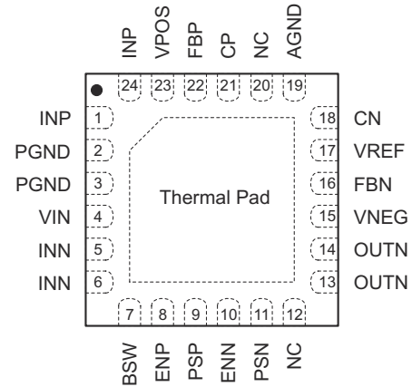
图 5-2. 24-pin VQFN Top View
