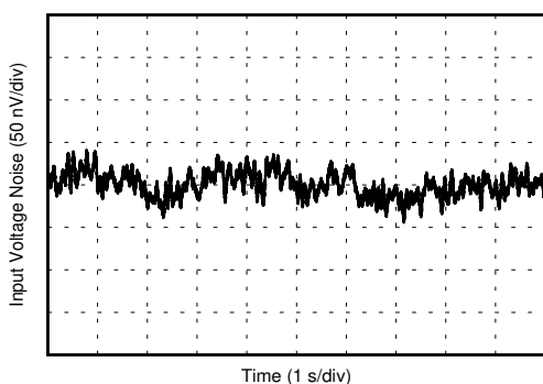
OPAx210 0.1Hz 至 10Hz 噪声
