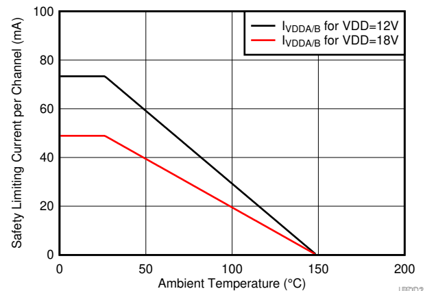
图 6-2. 根据 VDE 标准 限制电流的热降额曲线，DWK 封装
