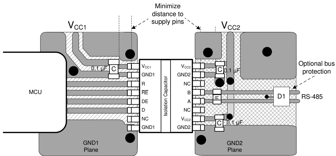
图 35. Layout Example
