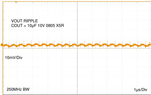
图 8-4. Output Ripple V_{OUT} = 1.2\text{ V}
