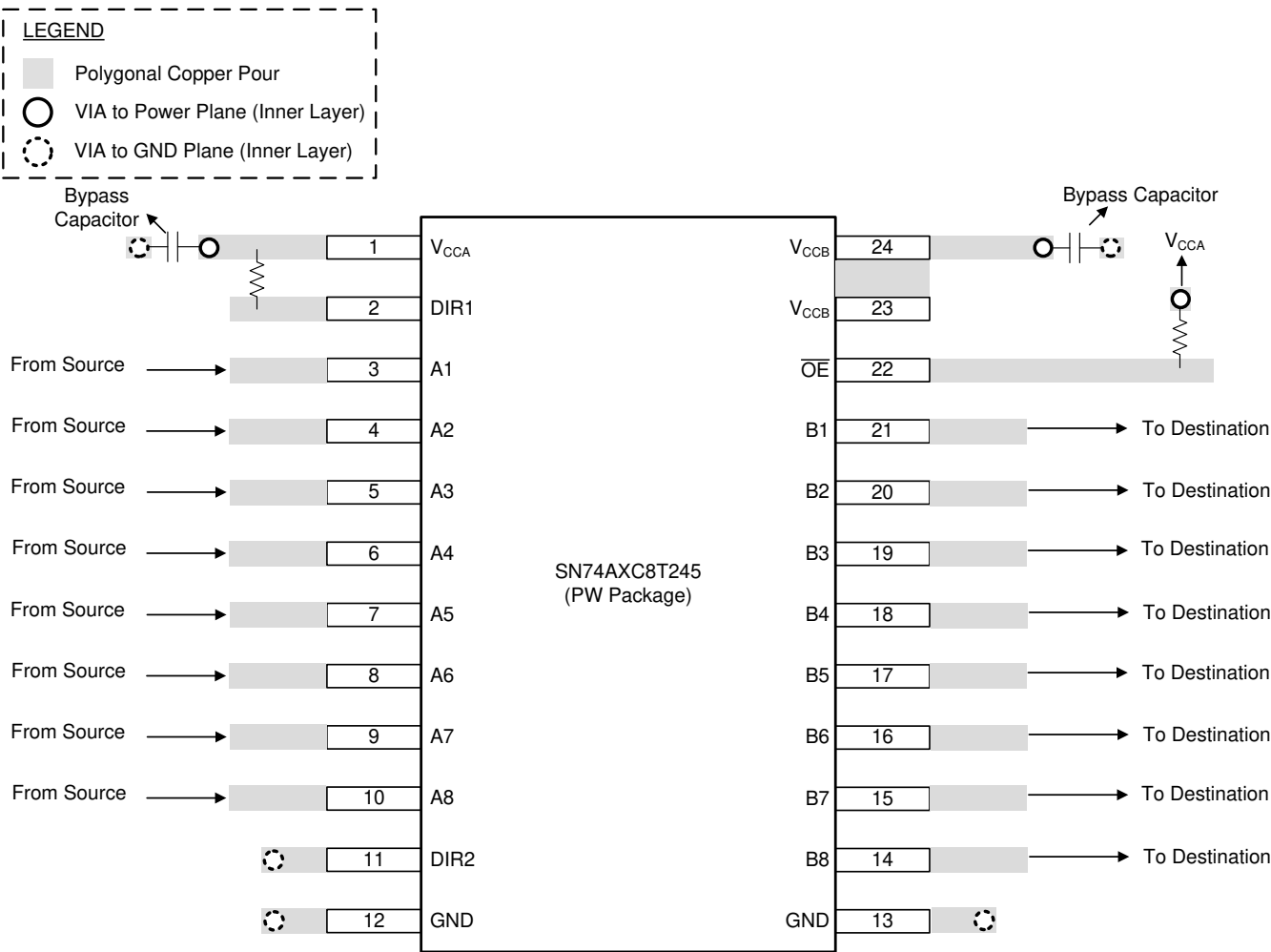
图 8-3. SN74AXC8T245 器件布局示例
