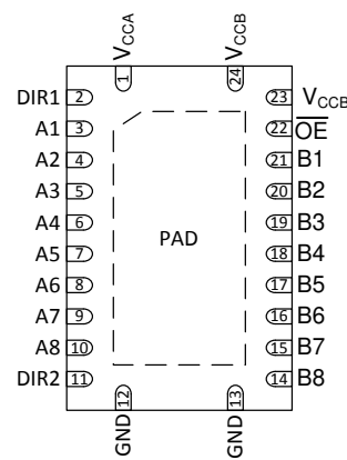
图 4-2. RHL 24 引脚 VQFN (俯视图)
