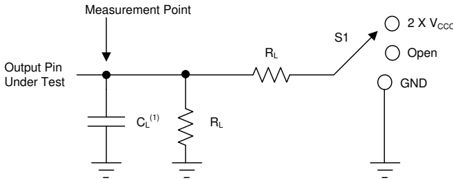
图 6-1. 负载电路
