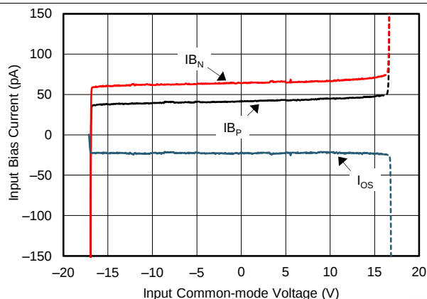
图 6. I_{\text{B}} 和 I_{\text{OS}} 与共模电压间的关系
