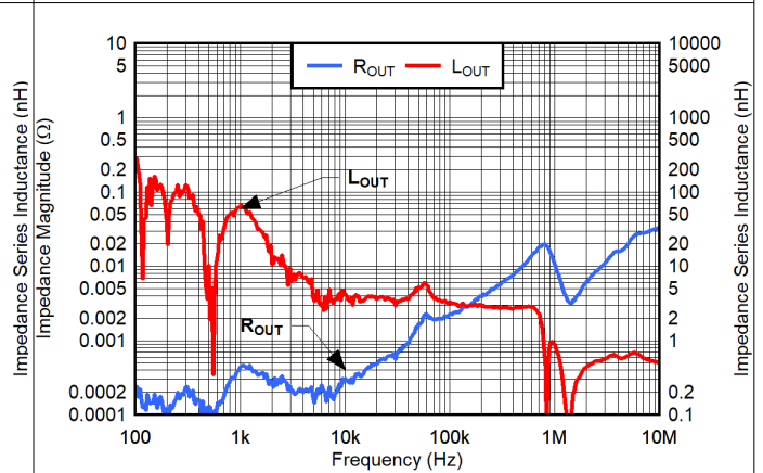
图 8-21. V_{IN} = 0.75\text{ V} , V_{BIAS} = 3\text{ V} , V_{OUT} = 0.5\text{ V} , CP\_EN = 0 , I_{OUT} = 1\text{ A}
