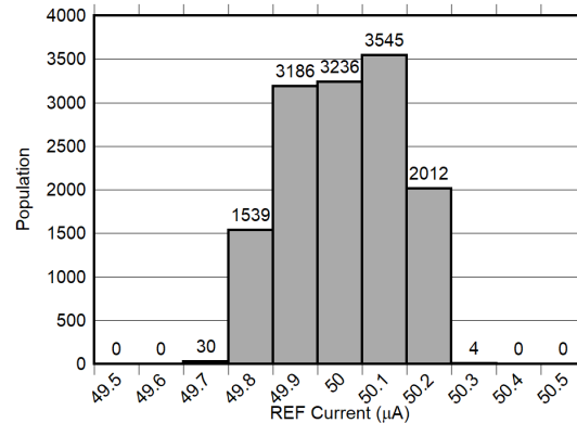
图 6-90. I_{REF} Distribution
