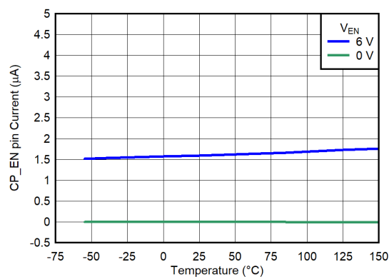
图 6-214. CP_EN Pin Current vs Temperature
