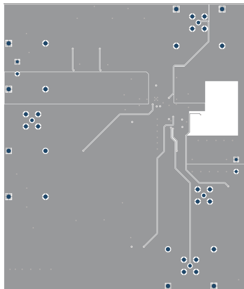
图 8-32. Layer 3 Routing
