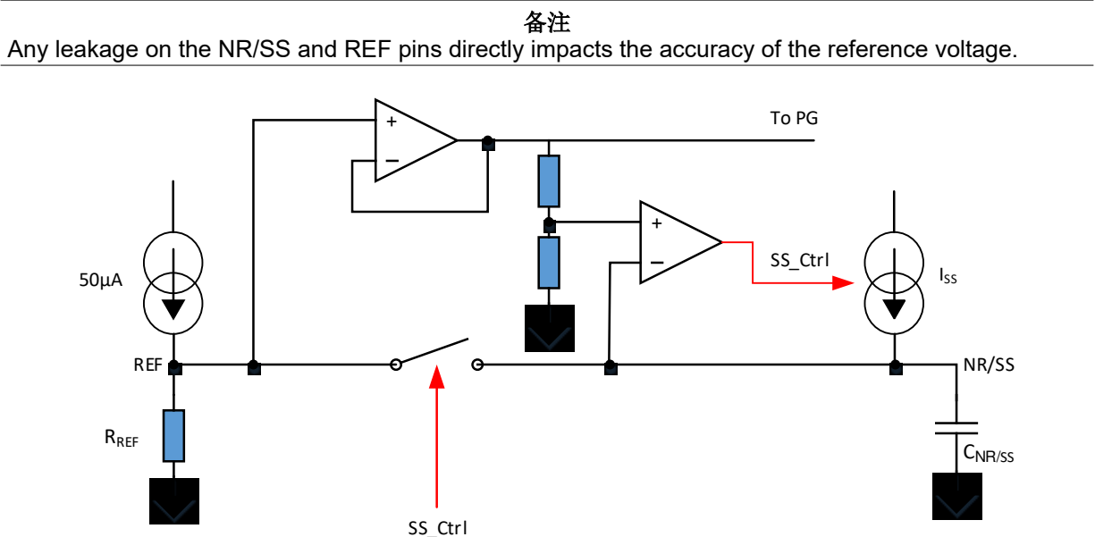
图 8-4. Simplified Soft-Start Circuit
