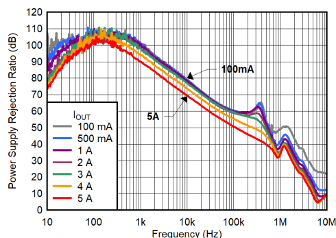
5A、1.2V IN 、0.9V OUT PSRR，已启用 CP
