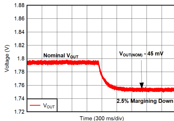
图 8-25. Margining Down
