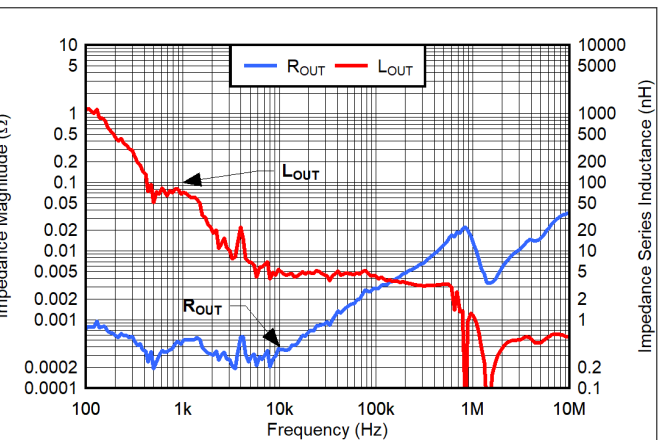
图 8-15. V_{IN} = 5.5\text{ V} , V_{OUT} = 5\text{ V} , V_{BIAS} = 8\text{ V} , CP\_EN = 0 , I_{OUT} = 500\text{ mA}
