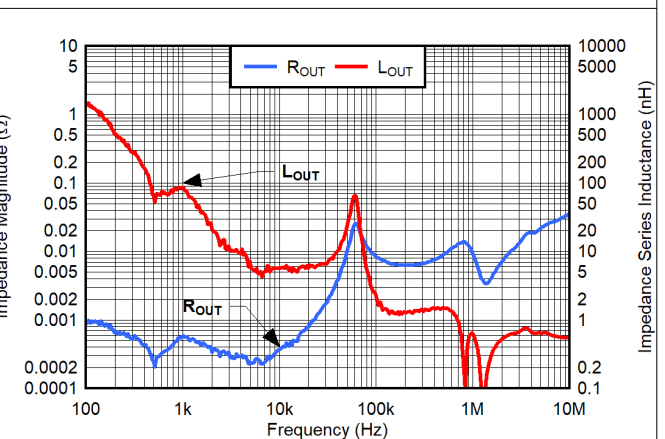
图 8-17. V_{IN} = 0.9\text{ V} , V_{BIAS} = 3\text{ V} , V_{OUT} = 0.5\text{ V} , CP\_EN = 0 , I_{OUT} = 4.6\text{ A}
