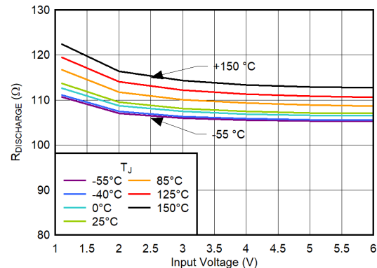
图 6-80. Output Discharge Resistor vs V_{IN}
