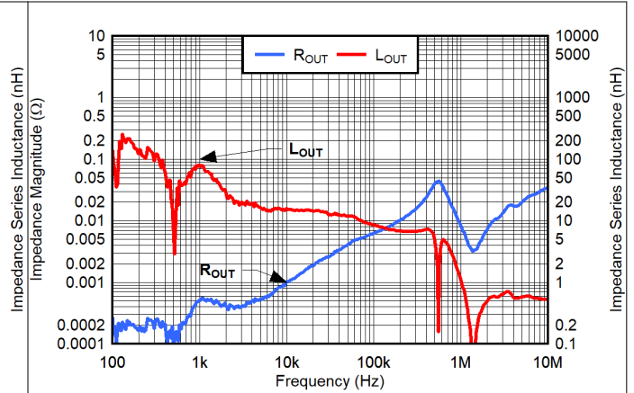
图 8-19. V_{IN} = 0.75\text{ V} , V_{BIAS} = 3\text{ V} , V_{OUT} = 0.5\text{ V} , CP\_EN = 0 , I_{OUT} = 100\text{ mA}
