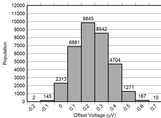
图 6-91. V_{OS} Distribution
