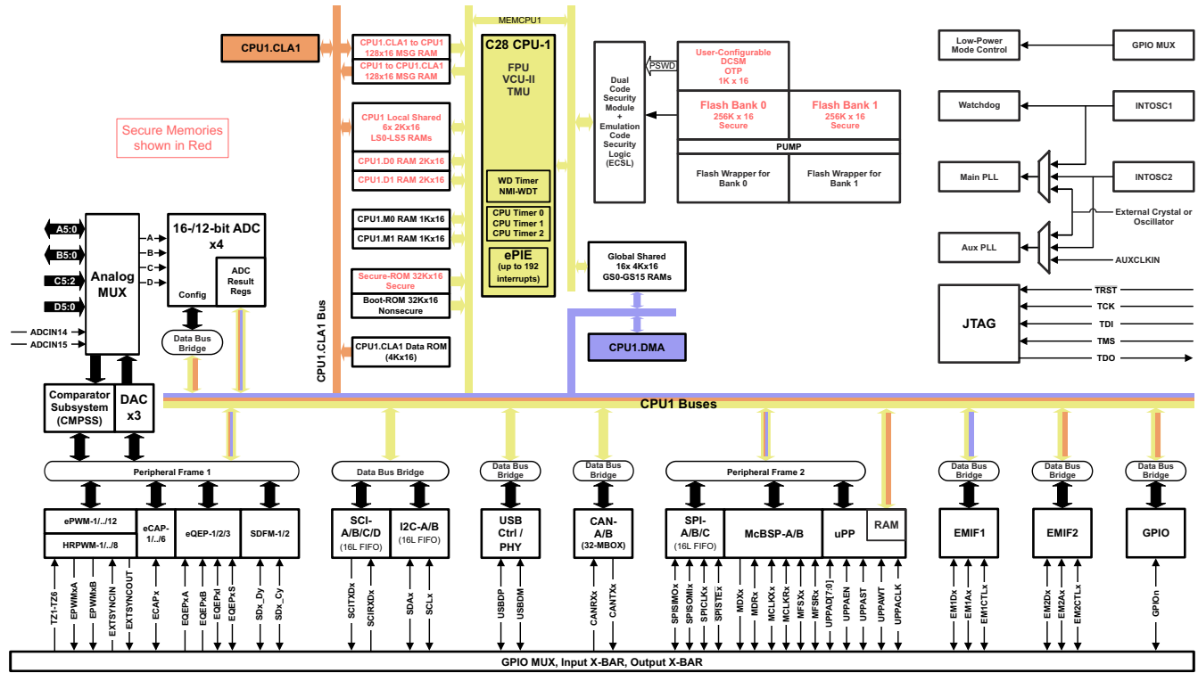
图 3-1. 功能方框图
