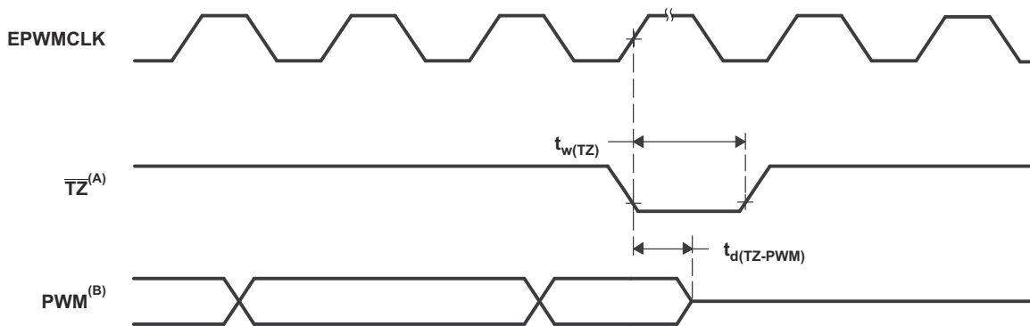
图 6-57. PWM Hi-Z 特性
