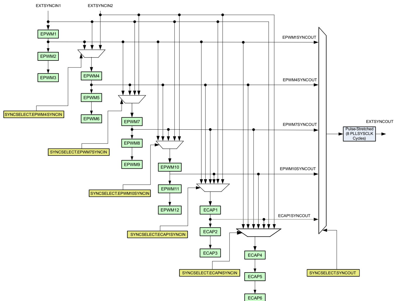
图 6-56. 同步链架构
