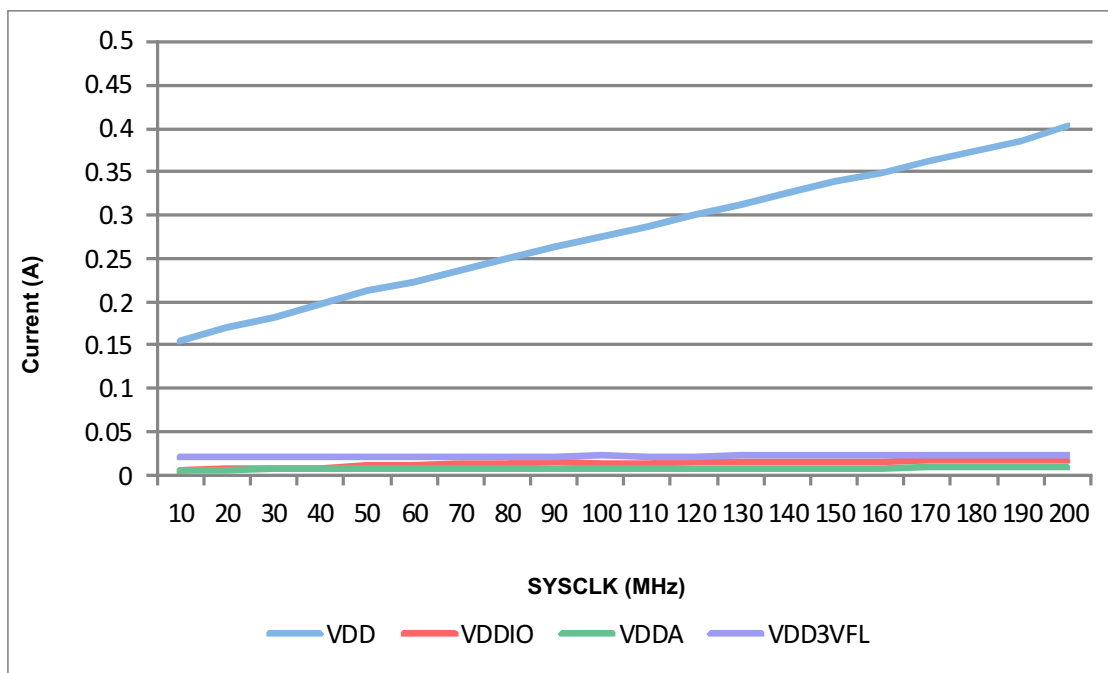
图 6-1. 工作电流与频率间的关系
