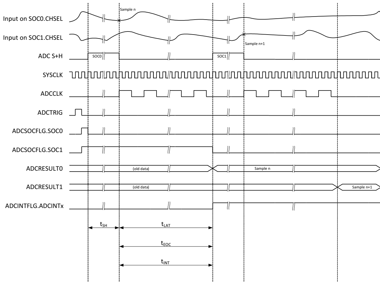
图 6-40. 16 位模式的 ADC 时序
