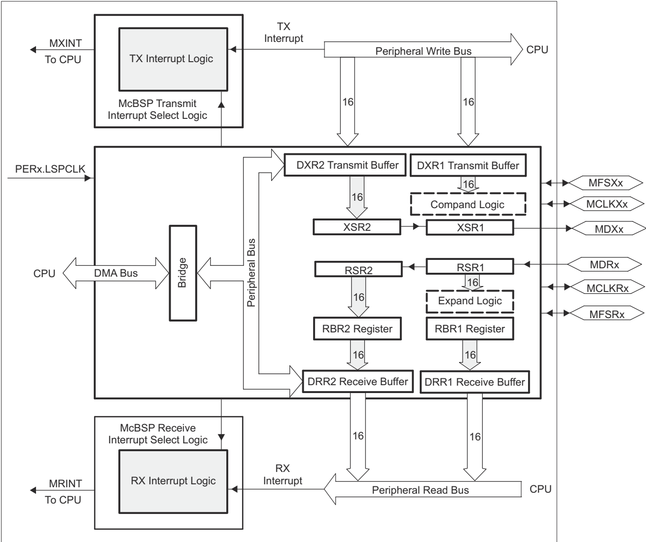
图 6-68. McBSP 方框图
