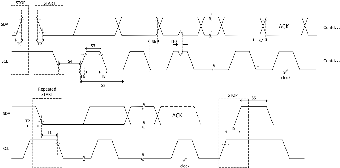
图 6-67. I2C 时序图
