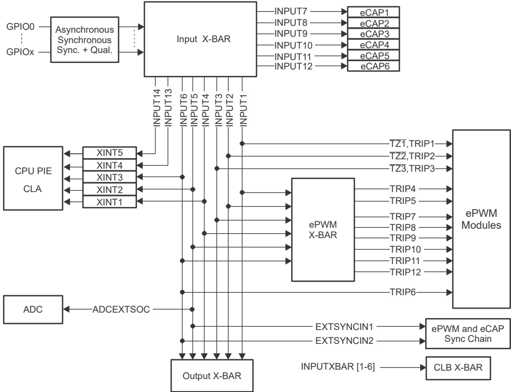
图 5-7. 输入 X-BAR
