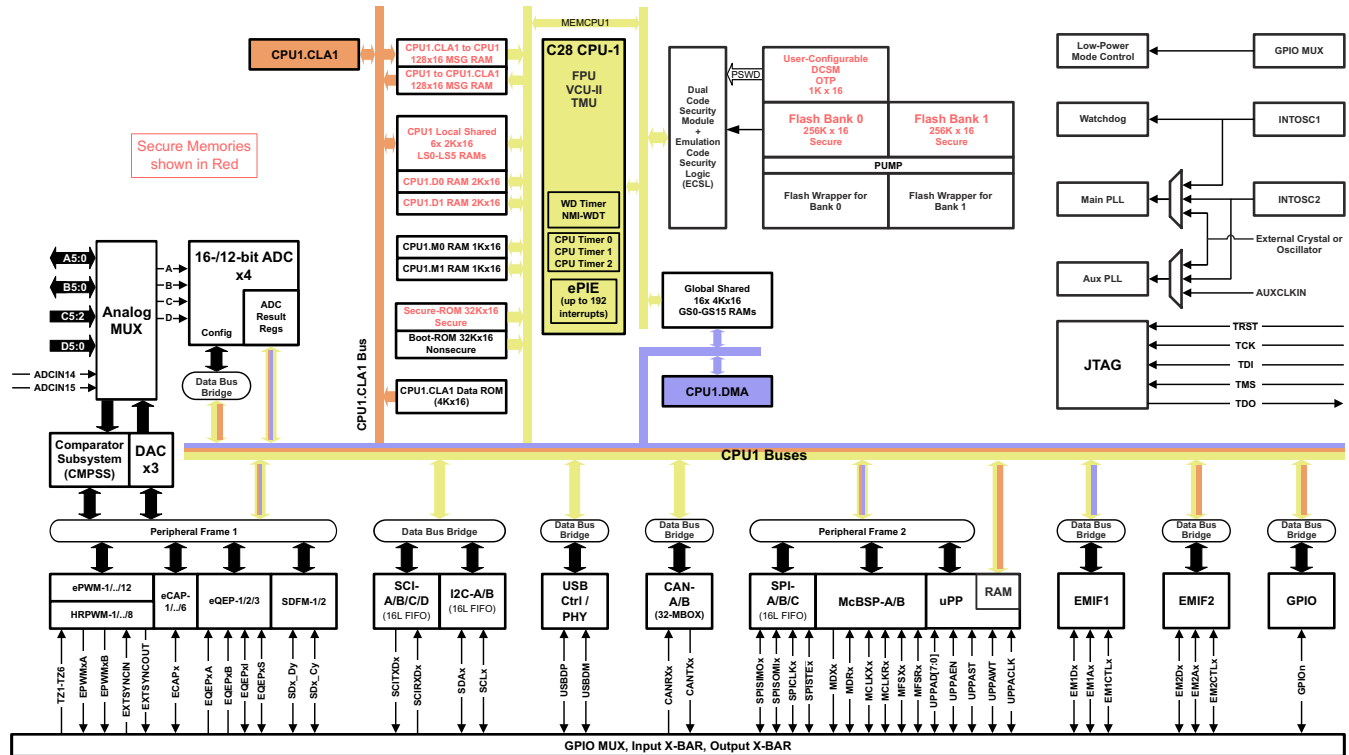
图 7-1. 功能方框图
