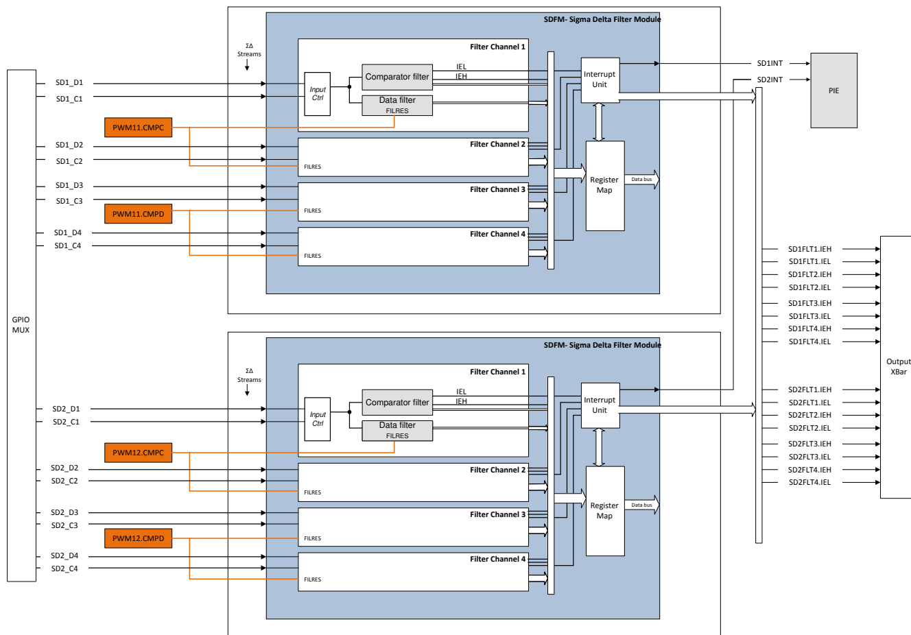
图 6-60. SDFM 方框图
