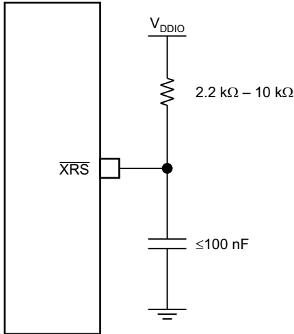
图 6-4. 复位电路
