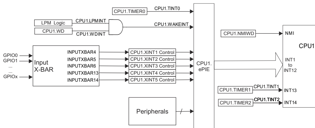
图 6-19. 外部和 ePIE 中断源
