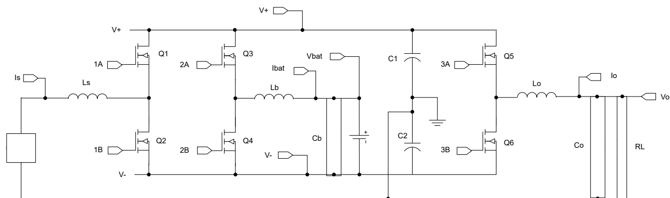
图 8-7. 三路转换在线 UPS 系统
