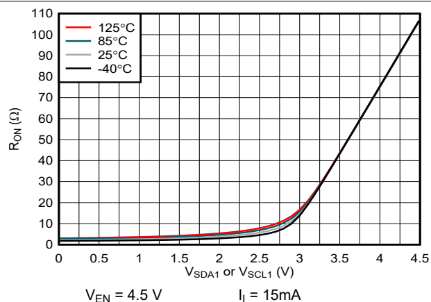
图 6-2. 导通电阻 ( R_{ON} ) 与输入电压间的关系 ( V_{SDA1} 或 V_{SCL1} )
