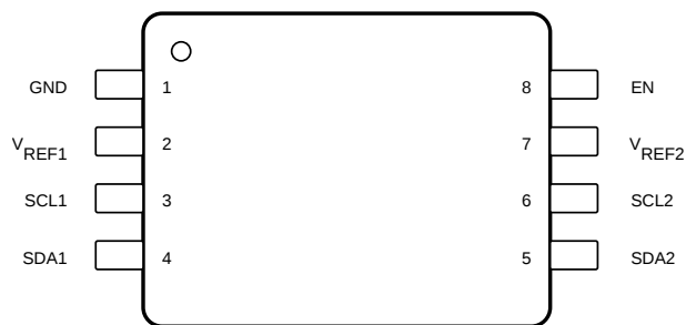
图 5-2. DCU 封装，8 引脚 VSSOP，顶视图
