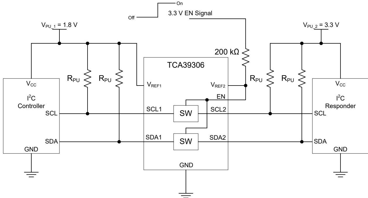
图 9-2. 典型应用电路 (开关使能控制)
