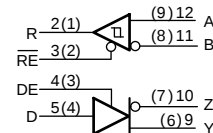
THVD1512 和 THVD1552 简化原理图
