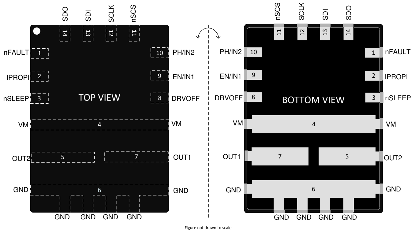
图 6-4. 采用 VQFN-HR (14) 封装的 DRV8243S-Q1 SPI 型号
