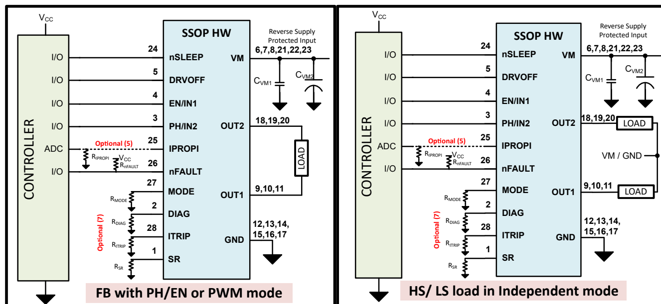
图 9-4. 典型应用原理图 - 采用 HVSSOP 封装的 HW 型号
