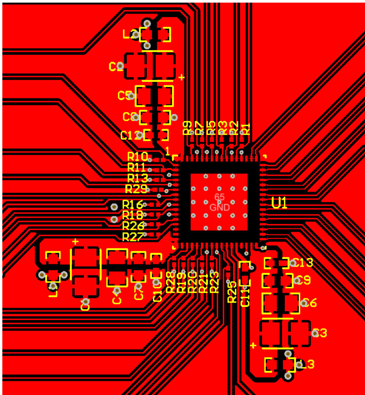
图 11-1. Layout Example
