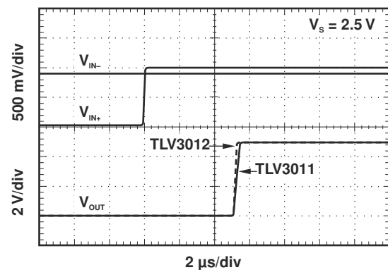
图 7-12. 传播延迟时间 ( t_{PHL} )
