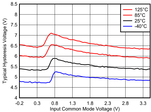
图 8-23. 迟滞电压与共模间的关系, 3.3\text{V}
