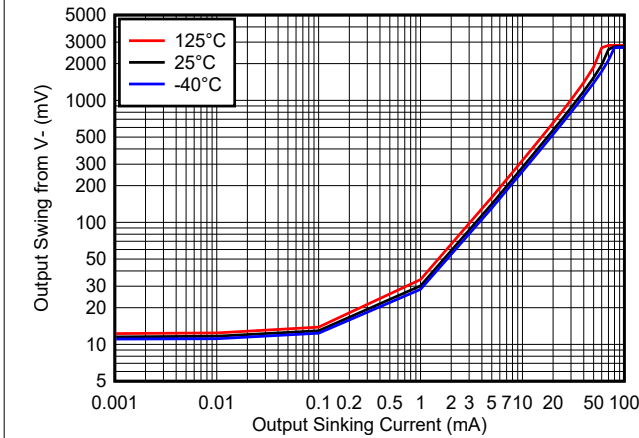
图 8-3. 输出摆幅与输出灌电流之间的关系 - 3.3V
