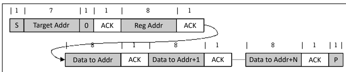
图 8-13. 多重写入
