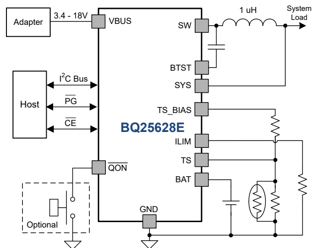
BQ25628E 简化版应用
