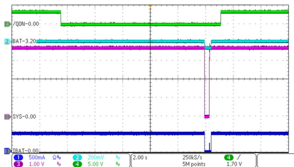
图 9-5. 充电禁用
