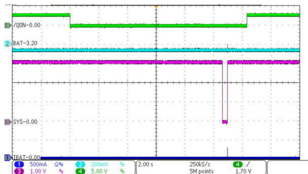
图 9-4. 充电启用
