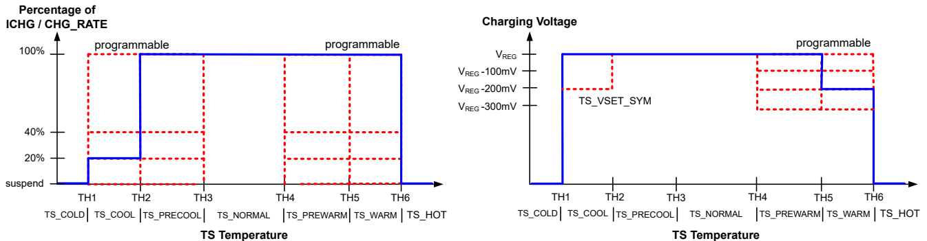
图 8-2. TS 充电值
