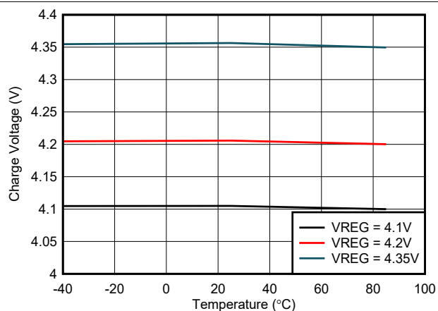
图 7-4. 充电电压精度与 VREG 设置间的关系
