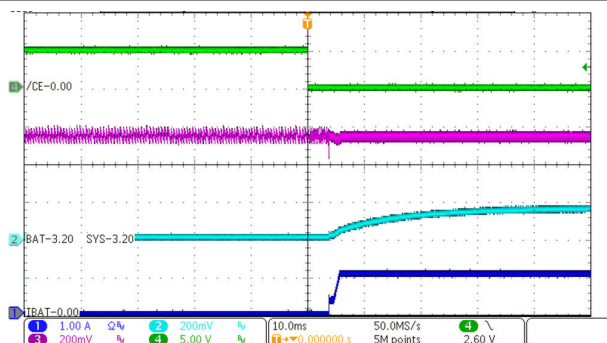
图 9-2. 在充电启用时上电
