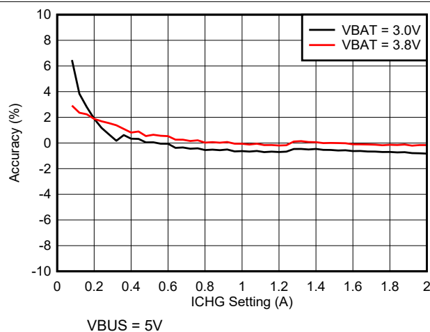
图 7-3. 充电电流精度与 ICHG 设置间的关系
