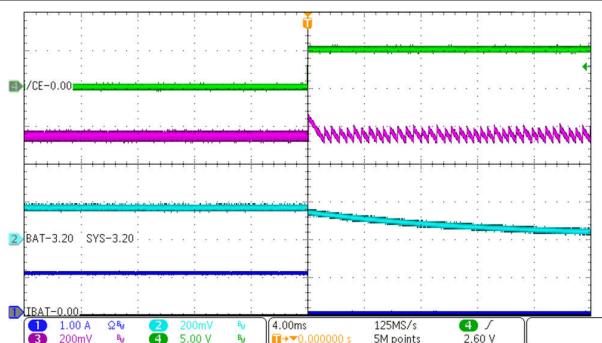
图 9-3. 断电
