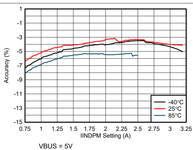
图 7-6. 输入电流调节精度与 IINDPM 设置间的关系
