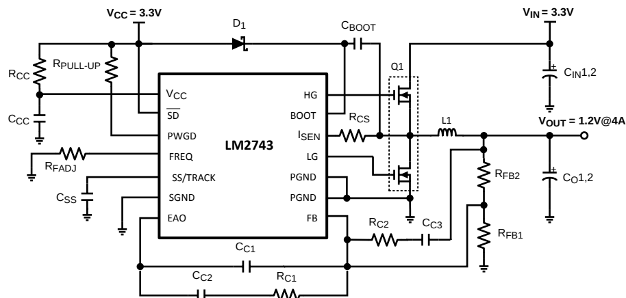
典型应用图
