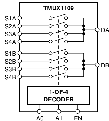
方框图
