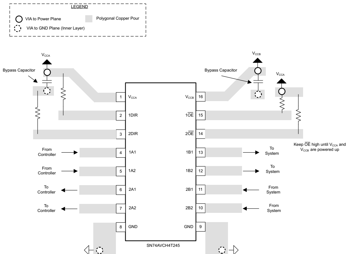
图 8-3. Layout Recommendation
