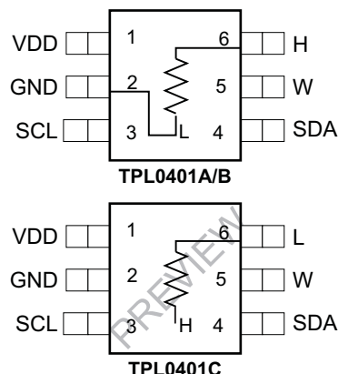
SC-70 DCK 封装 (顶视图)
