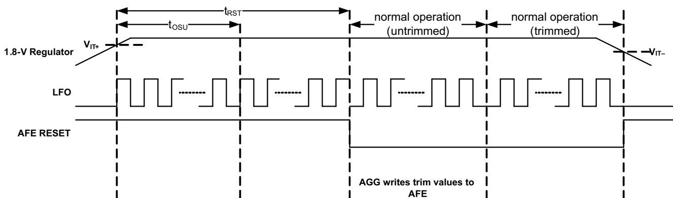
图 8-2. POR Timing Diagram
