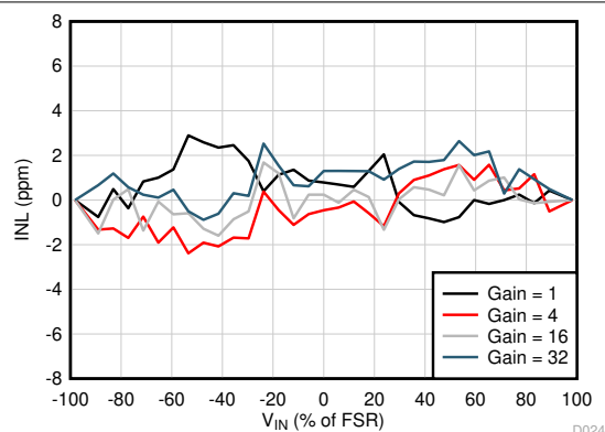
图 7-21. ADC1 INL vs V_{IN}
