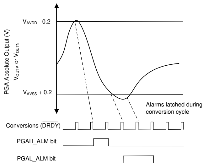
图 9-11. PGA Absolute Alarm
