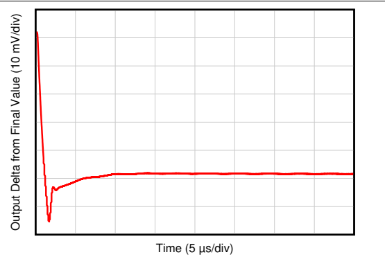
图 7-34. 小信号阶跃响应
