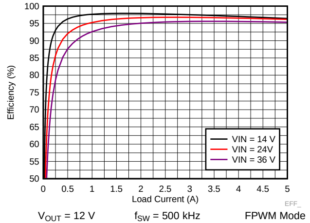
图 40. LM73605 Efficiency
