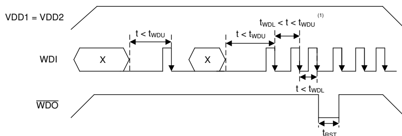
图 6-1. Timing Diagram
