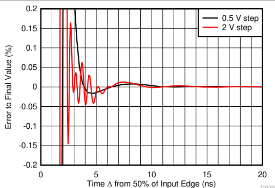
图 6-27. 小信号和大信号阶跃响应
