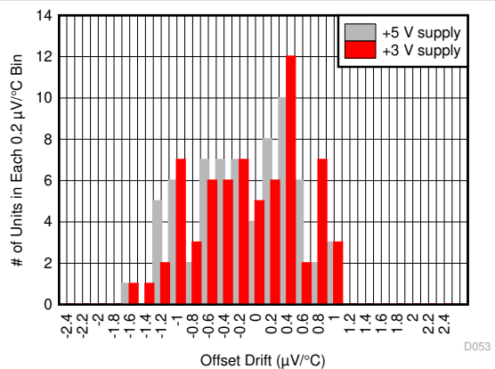
图 6-51. 输入失调电压随温度变化的情况
