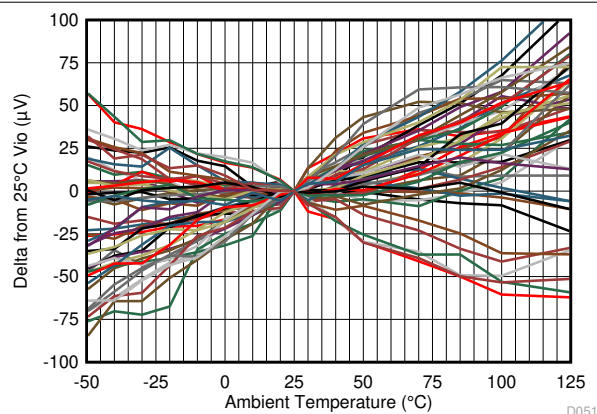
图 6-49. 输入失调电压
