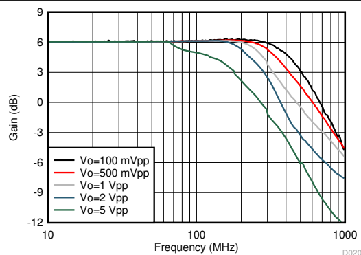
图 6-20. 频率响应与 V_{opp} 之间的关系
