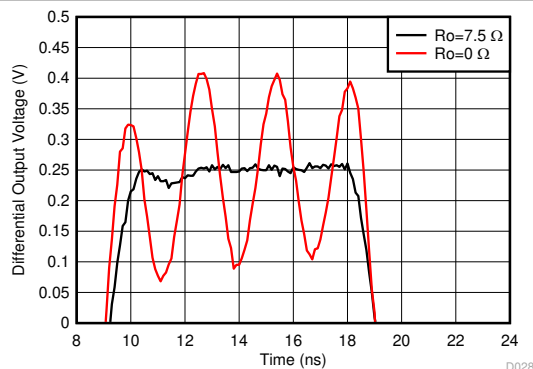
图 6-28. 容性负载的阶跃响应
