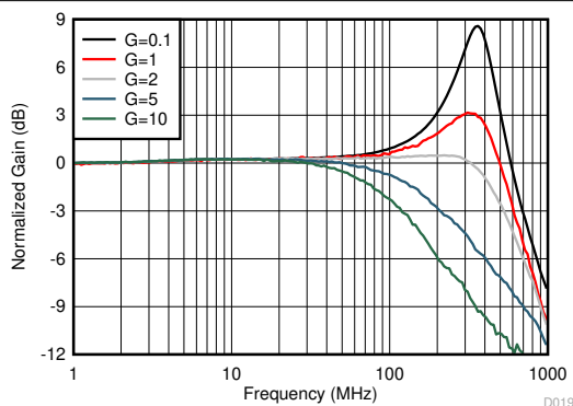
图 6-19. 小信号频率响应与增益间的关系
