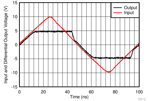
图 6-12. 过驱恢复性能
