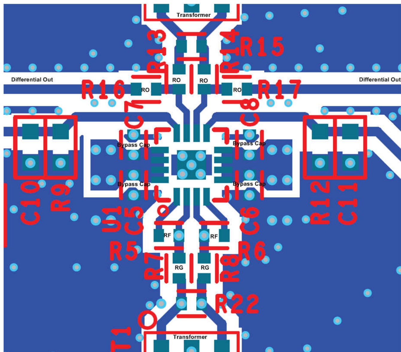
图 9-6. 布局示例
