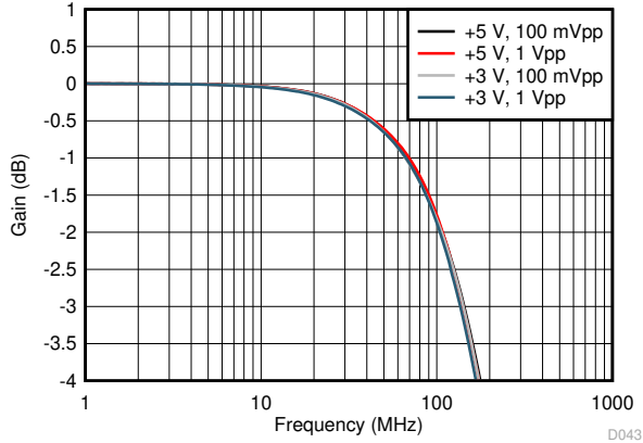
图 6-43. 共模，小信号和大信号响应（ V_{ocm} 引脚驱动）
