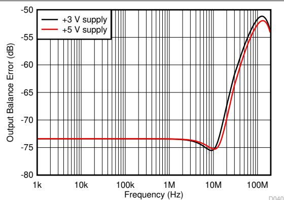
单端输入至差分输出，增益为 2（请参阅图 7-1），使用 1% 电阻器进行仿真，最坏情况失配
