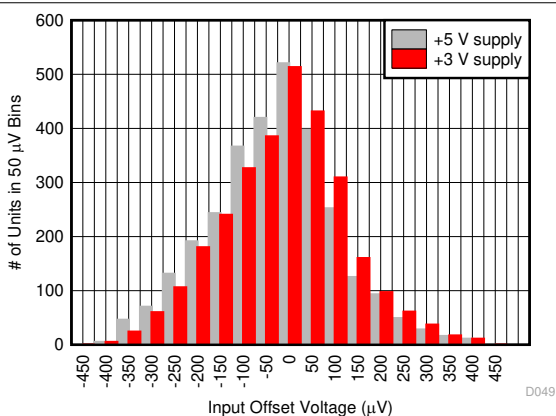
图 6-49. 输入失调电压
