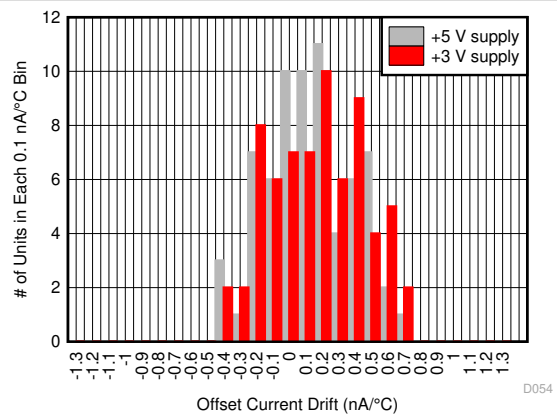
图 6-52. 输入失调电流随温度变化的情况
