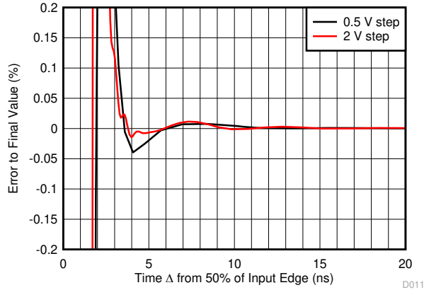
图 6-11. 小信号和大信号阶跃稳定时间
