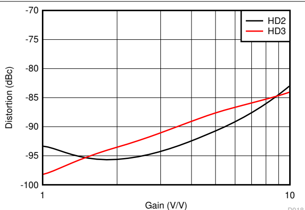
图 6-18. 谐波失真与增益间的关系
