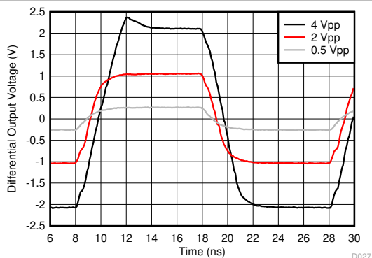
图 6-27. 小信号和大信号阶跃响应
