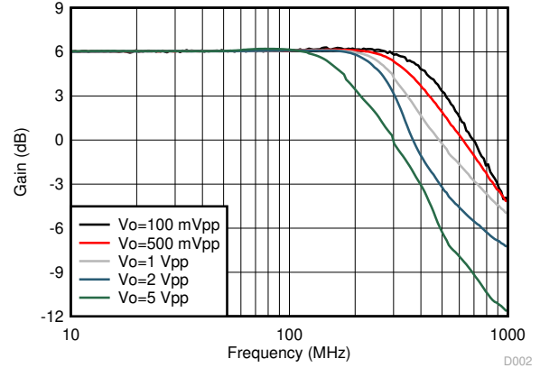
图 6-2. 频率响应与 V_{opp} 之间的关系
