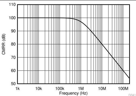
共模输入至差分输出，增益为 2 的仿真
