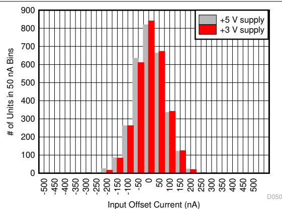
图 6-50. 输入失调电流
