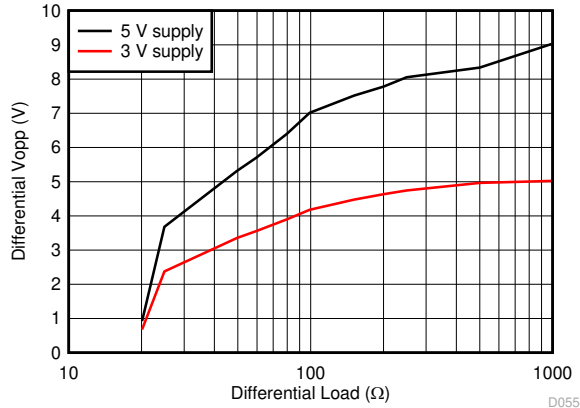
图 6-55. 最大 V_{opp} 与 R_{load} 之间的关系
