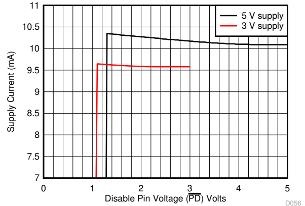
图 6-56. 电源电流与 \overline{PD} 电压之间的关系
