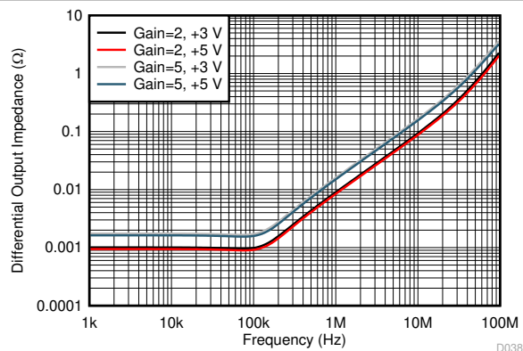
单端输入至差分输出，仿真差分输出阻抗，（闭环）增益为 2 和 5，请参阅图 7-1
