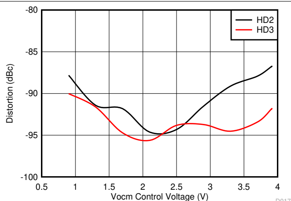
图 6-17. 谐波失真与 V_{ocm} 之间的关系
