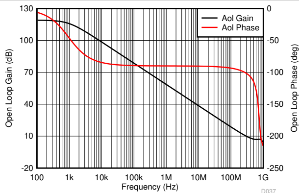
图 6-37. 主放大器差分开环增益和相位与频率之间的关系
