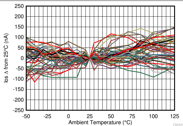
图 6-50. 输入失调电流
