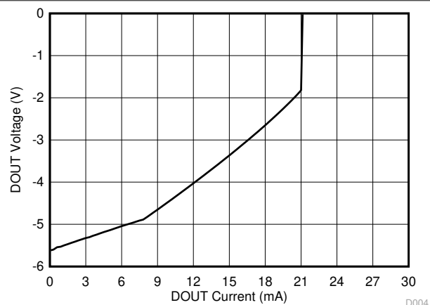
图 5-4. 驱动器 VOL 与负载电流间的关系
