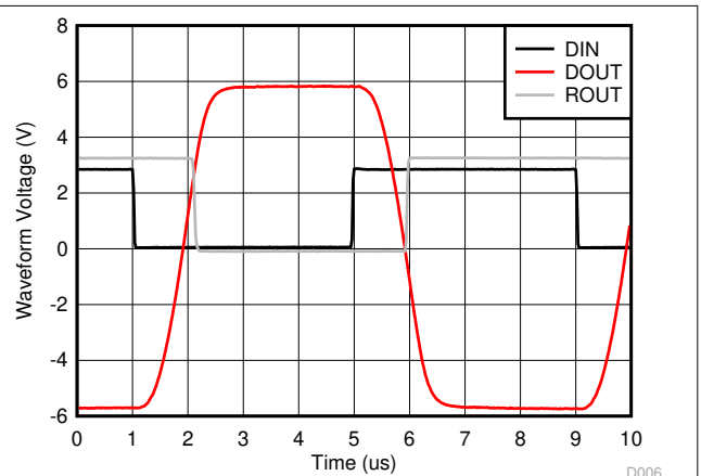
图 8-3. 1nF 负载、 V_{CC} = 3.3V 、数据速率 250kbit/s 时的环回波形
