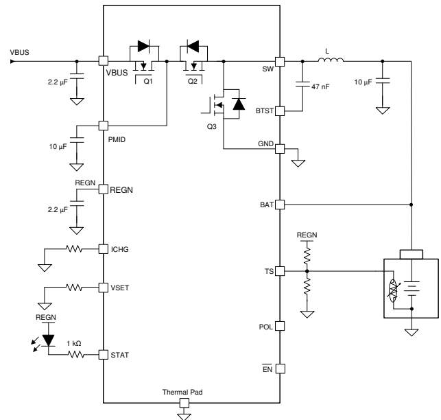
简化版应用
