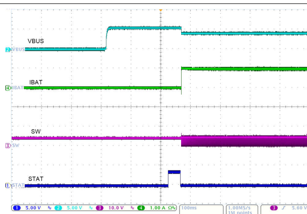
图 10-3. 充电周期
