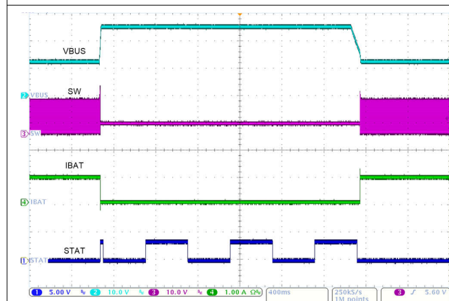
图 10-2. 从 VBUS 上电
