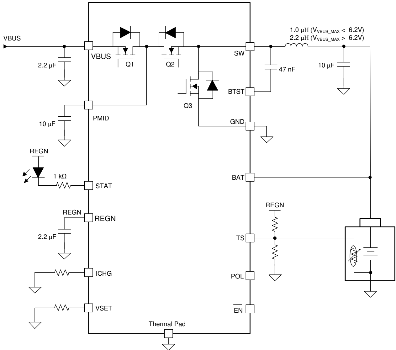
图 10-1. 典型应用图
