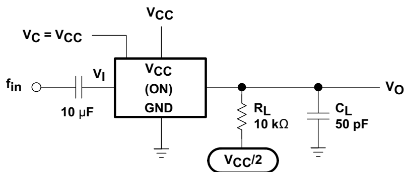
图 6-11. Amplitude-Distortion Rate
