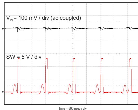
图 7-9. Input Voltage Ripple, I_{OUT} = 800 \text{ mA}
