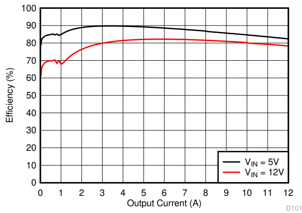
图 7-2. Efficiency
