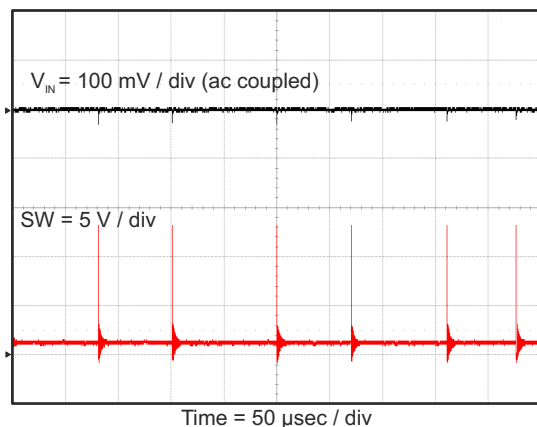
图 7-8. Input Voltage Ripple, I_{OUT} = 10 \text{ mA}
