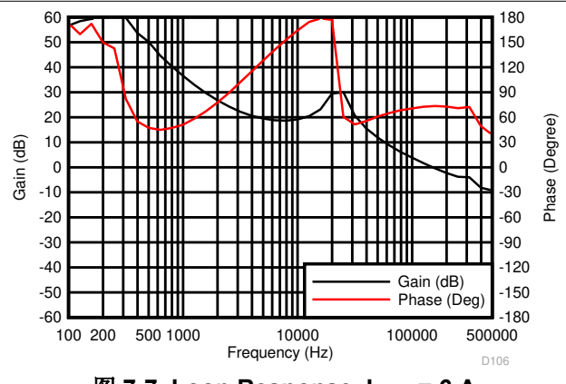
图 7-7. Loop Response, I_{OUT} = 6\text{ A}
