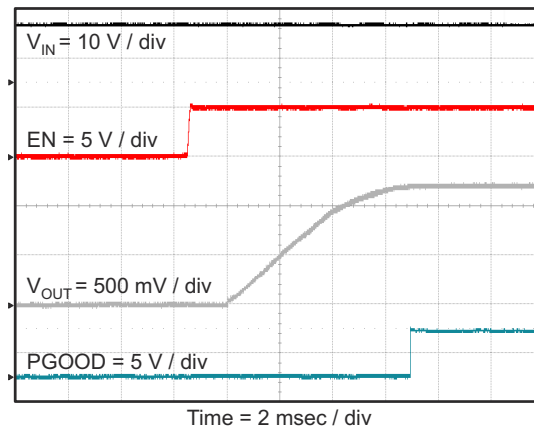
图 7-15. Start Up Relative to EN Rising
