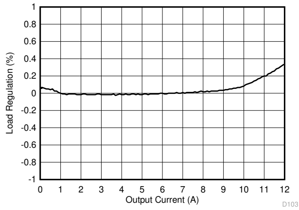
图 7-4. Load Regulation, V_{IN} = 5\text{ V}
