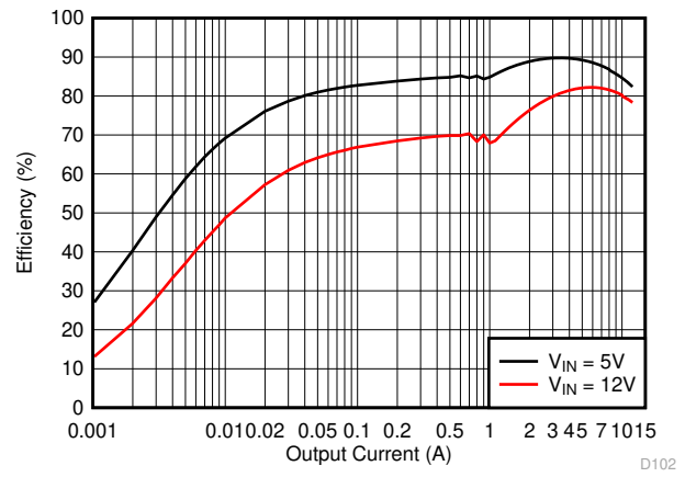
图 7-3. Light Load Efficiency
