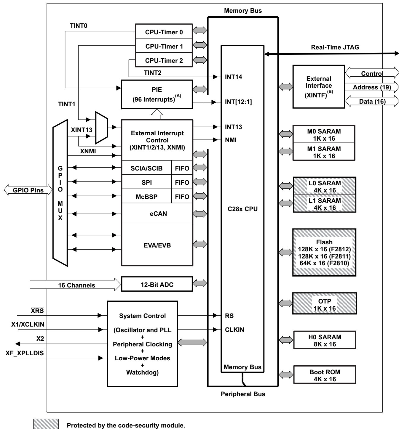
图 1-1. 功能方框图
