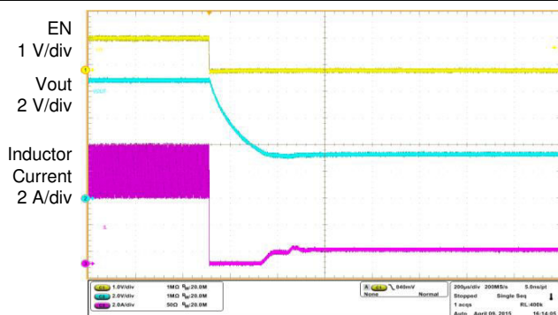
图 8-6. Shutdown Waveforms
