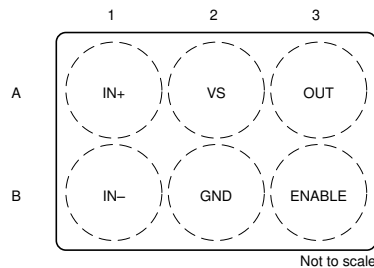
图 5-2. YFD 封装 6 引脚 DSBGA 顶视图
