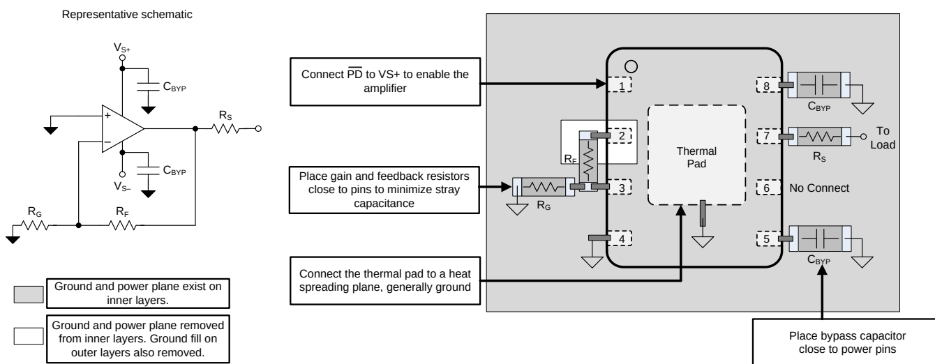
图 18. Layout Recommendation
